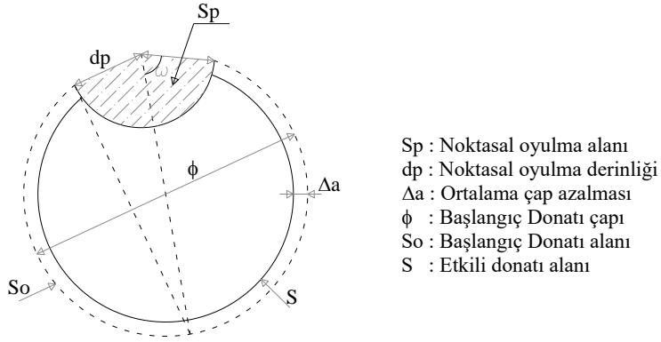
Şekil 5. Korozyon etkisi altındaki donatı enkesiti
